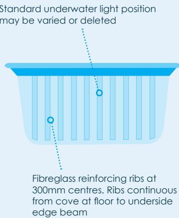
END ELEVATION
